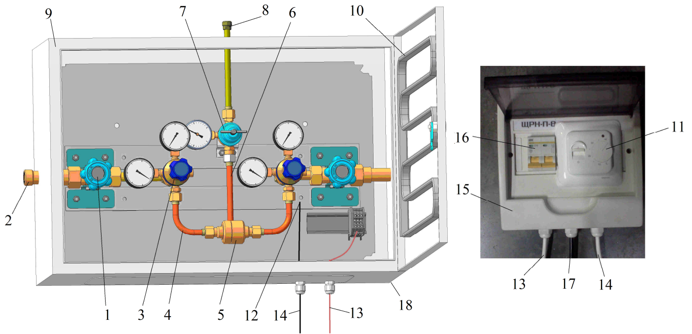
Рис.1а Щит автопереключения газовых рампов закрытого типа в термобоксе исп. ДЖЕТ 653 20 00 00.
